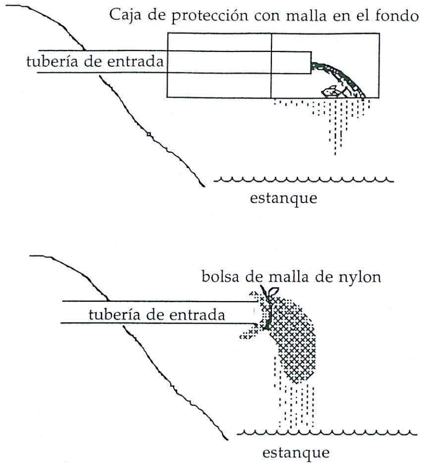
Figura 4: Caja de filtración y bolsa de malla de nylon pueden ser utilizadas para filtrar el agua que entra al estanque por medio de tuberías.
